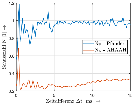
Abbildung 8: Schusszahlen in Abhängigkeit von Zeitdifferenzen
