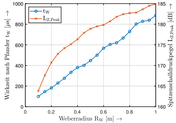
Abbildung 5: Wirkzeit und Spitzenschalldruck in Abhängigkeit des Weberradius
