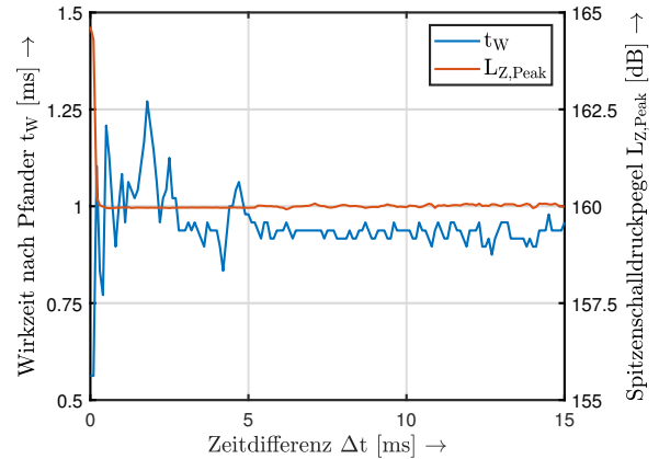
Abbildung 9: Wirkzeit und Spitzenschalldruckpegel in Abhängigkeit von Zeitdifferenzen
