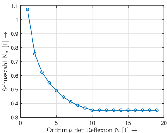
Abbildung 11: Schusszahlen nach dem AHAAH-Modell in Abhängigkeit der Reflexionsordnung
