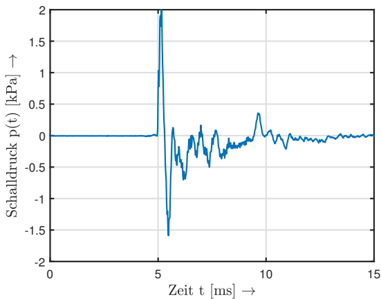
Abbildung 4: Schalldruckzeitverlauf des Waffenknalls
