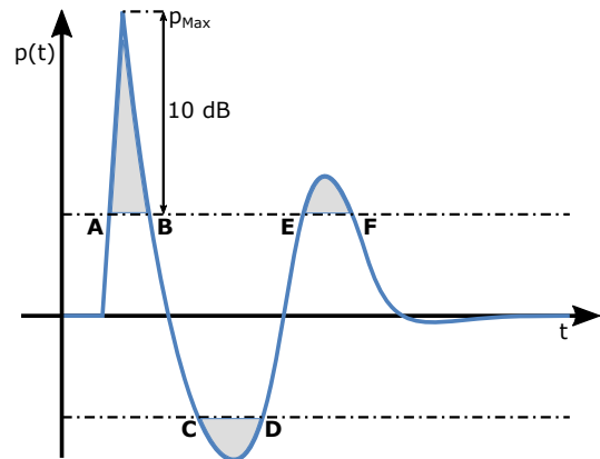
Abbildung 2: Bestimmung der Wirkzeit [1]
