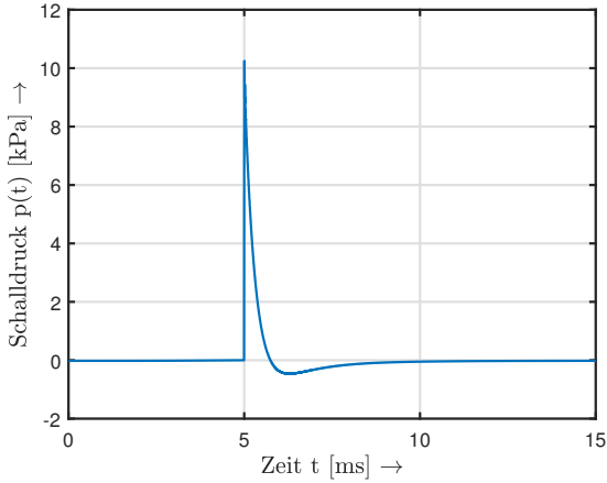
Abbildung 3: Schalldruckzeitverlauf des Weberknalls
