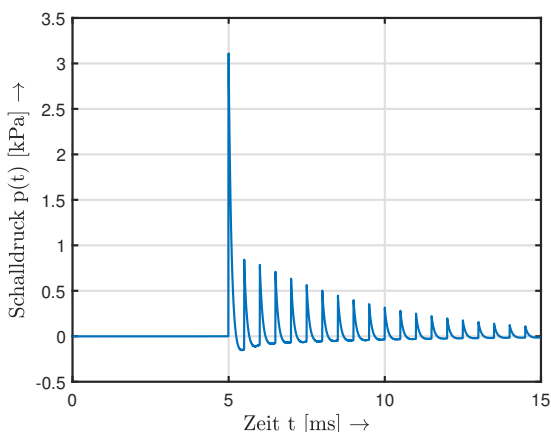
Abbildung 10: Weberknall mit künstlichen Reflexionen
