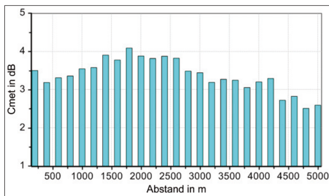
Bild 8 C_{\text{met}} nach Süden.
