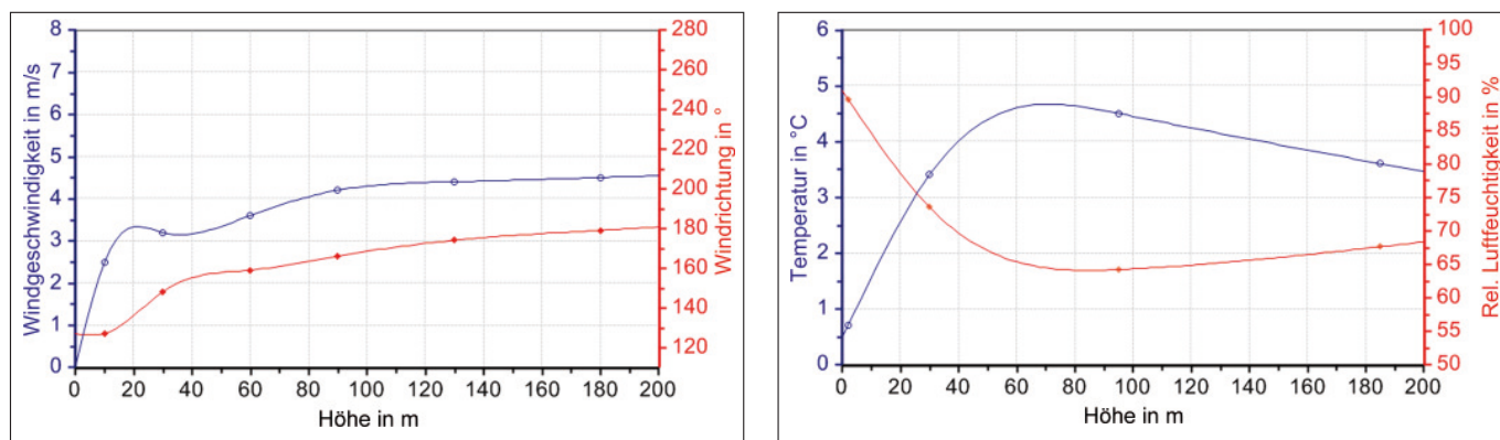
Bild 2 Darstellung einer stundenspezifischen Profilprognose gegenüber der Höhe; links: Windgeschwindigkeit blau und Windrichtung rot, rechts: Temperatur blau, relative Luftfeuchtigkeit rot
