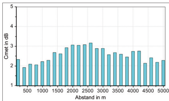
Bild 9 C_{\text{met}} nach Norden.
