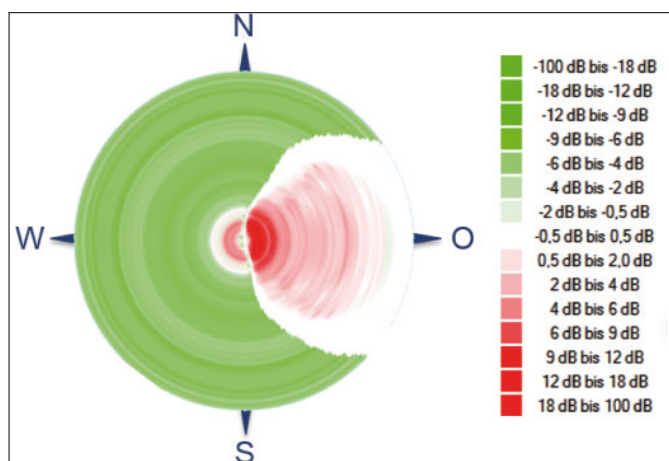
Bild 6 Lärmrose mit einer Abstandsklassierung von 50 bis 5 000 m, einer Winkelklassierung von 1° und einer Pegelklassierung, wie rechts dargestellt.
