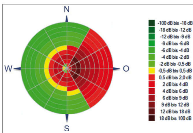
Bild 5 Lärmrose mit einer Abstandsklassierung von 200 bis 2 000 m, einer Winkelklassierung von 30° und einer Pegelklassierung, wie rechts dargestellt.
